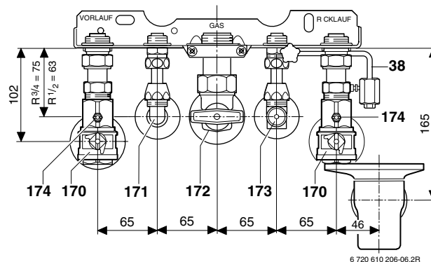
Bild 8 Montageanschlussplatte mit Unterputz-Installation (fertig montiert)
