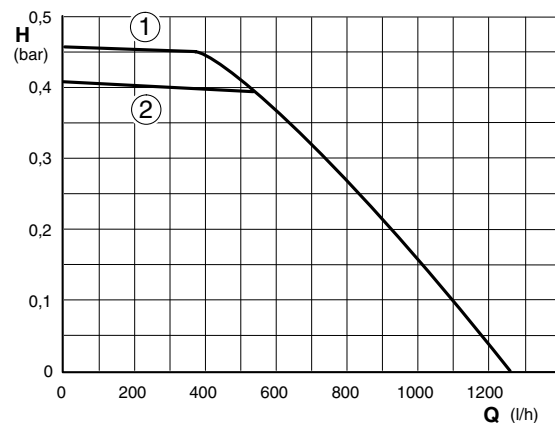
Bild 33 Konstantdruck
