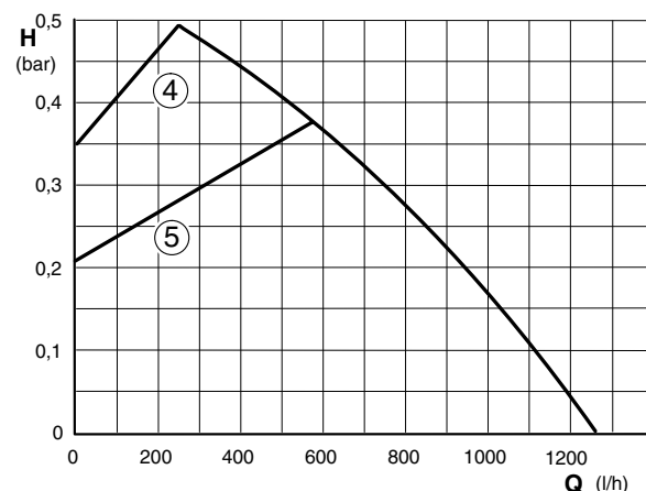
Bild 34 Proportionaldruck
